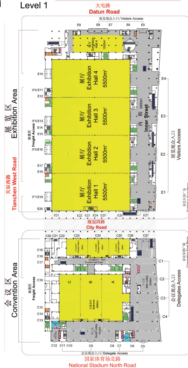
一层平面图 Level 1
